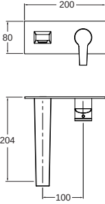
Set da incasso CS 237-238 pag. 14-15 Unterputz-Einbaukörper CS 237-238 Seite 14-15 Mécanisme encastré CS 237-238 page 14-15 Concealed body CS 237-238 page 14-15 Cuerpo de empotrado CS 237-238 página 14-15 Встраиваемый компонент CS 237-238 стр. 14-15
