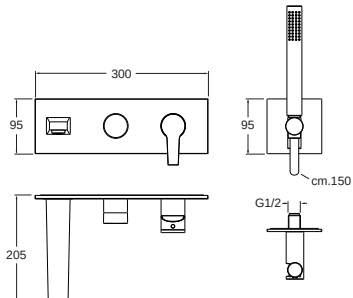
Set da incasso CS 147 pag. 14 Unterputz-Einbaukörper CS 147 Seite 14 Mécanisme encastré CS 147 page 14 Concealed body CS 147 page 14 Cuerpo de empotrado CS 147 página 14 Встраиваемый компонент CS 147 стр. 14
