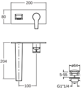
Set da incasso CS 237-238 pag. 14-15 Unterputz-Einbaukörper CS 237-238 Seite 14-15 Mécanisme encastré CS 237-238 page 14-15 Concealed body CS 237-238 page 14-15 Cuerpo de empotrado CS 237-238 página 14-15 Встраиваемый компонент CS 237-238 стр. 14-15
