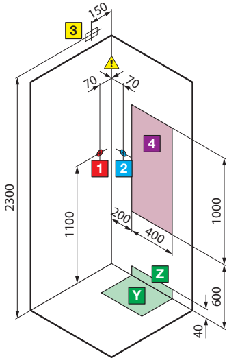
versión izquierda / versão esquerda versión derecha / versão direita para modelo A100x80 - A120x80
