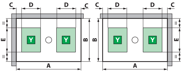
S INSTALACIÓN A MANO IZQUIERDA INSTALAÇÃO ESQUERDA
