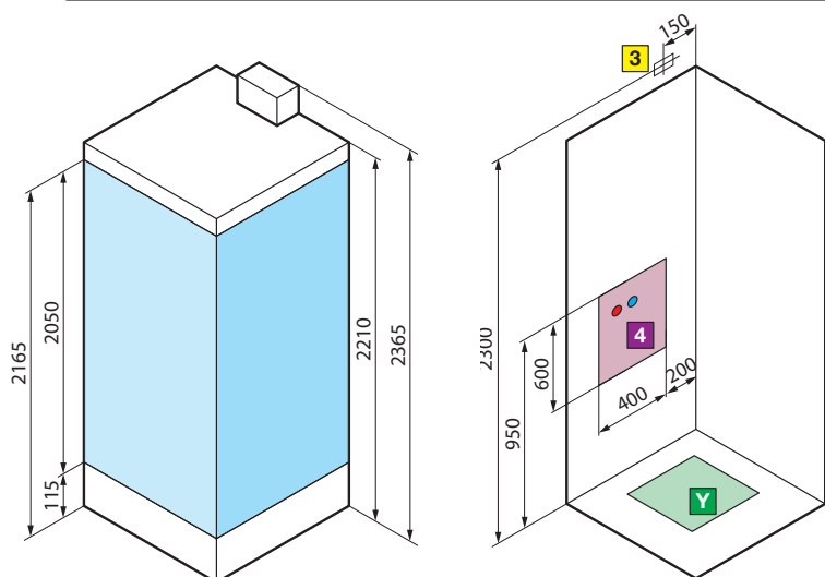
para modelos GF/A80 - GF/A90 - R90
