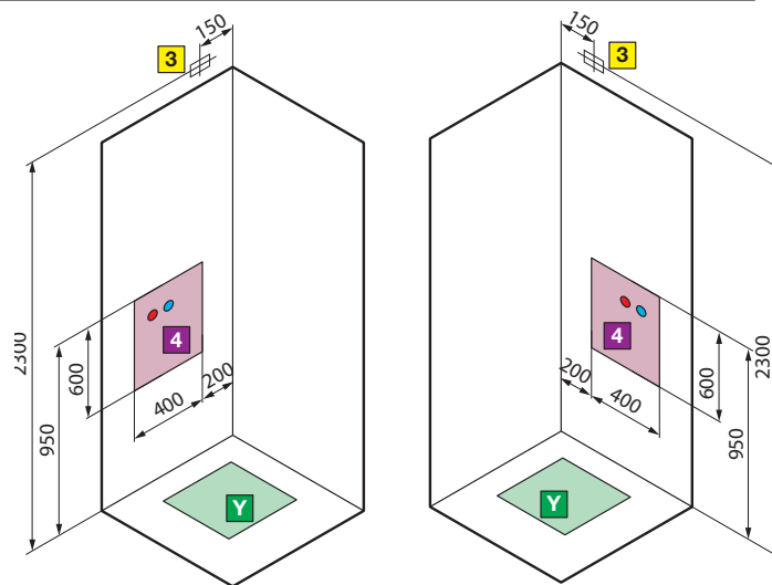
versión izquierda / versão esquerda | versión derecha / versão direita para modelos A100x80 - 2P120x80 - 2P120x90
