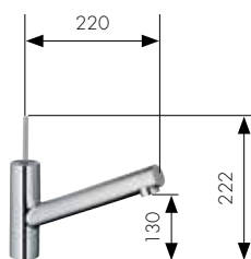
Miscelatore da cucina monocomando con maniglia cilindrica # 10801000
