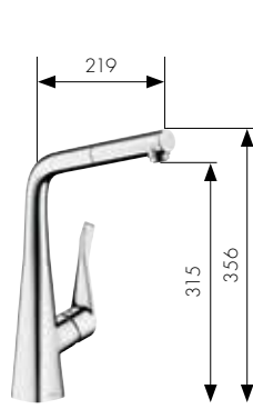
Miscelatore da cucina monocomando con erogazione estraibile # 14821, -000, -800
