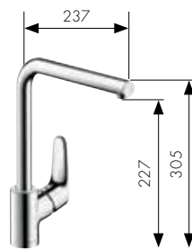
Miscelatore da cucina monocomando con bocca orientabile (erogatore a L) # 31817, -000, -800
