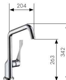
Miscelatore da cucina monocomando con bocca orientabile # 39850, -000, -800
