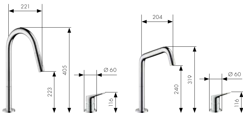
Miscelatore da cucina monocomando a 2 fori con doccetta estraibile # 34822, -000, -800
