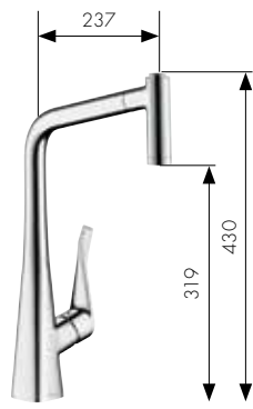
Miscelatore da cucina monocomando con doccetta estraibile # 14820, -000, -800
