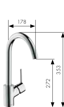
Miscelatore da cucina monocomando con bocca alta orientabile # 14870, -000, -800
