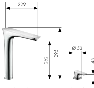
Miscelatore da cucina monocomando a 2 fori # 15812, -000, -800
