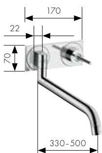
Miscelatore da cucina monocomando da incasso # 38815, -000, -800 Corpo incasso senza figura) # 13622180
