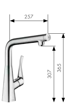
Miscelatore da cucina Select # 14883, -000, -800
