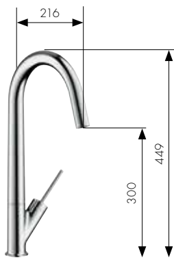
Miscelatore da cucina monocomando con bocca orientabile # 10822, -000, -800
