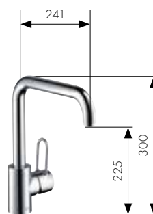
Miscelatore da cucina con bocca orientabile # 1485000 con valvola di arresto (senza figura) # 14855000
