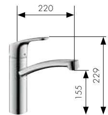
Miscelatore da cucina monocomando # 31806, -000, -800
