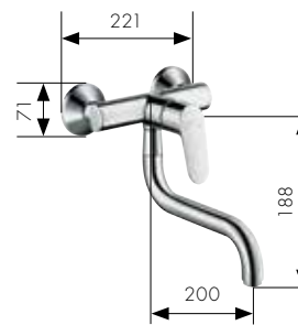
Miscelatore da cucina monocomando a parete # 31825000
