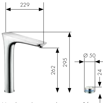
Miscelatore da cucina elettronica a 2 fori # 15805, -000, -800
