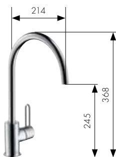
Miscelatore da cucina monocomando con erogazione orientabile # 38830, -000, -800
