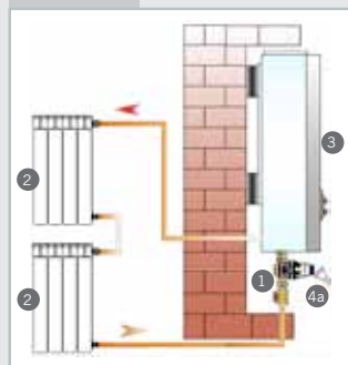
INSTALLAZIONE 4
