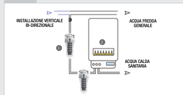
INSTALLAZIONE
