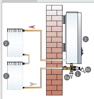
INSTALLAZIONE 2
