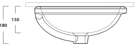
lavabo sottopiano da incasso ovale 50 installazione su piano. Kit di fissaggio incluso.
