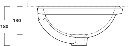
lavabo sottopiano da incasso rotondo 33 installazione su piano. kit di fissaggio incluso.
