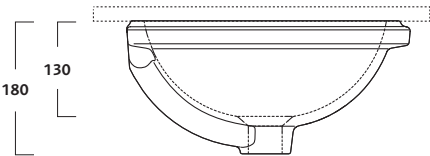
lavabo sottopiano da incasso ovale 42 installazione su piano. Kit di fissaggio incluso.
