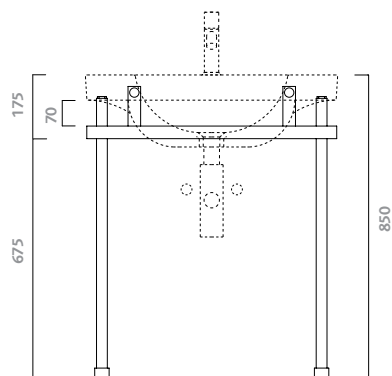
composizione 4108 struttura in ottone cromato con lavabo rettangolare 70 (41022)
