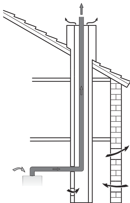
Tipologia di scarico "B"
