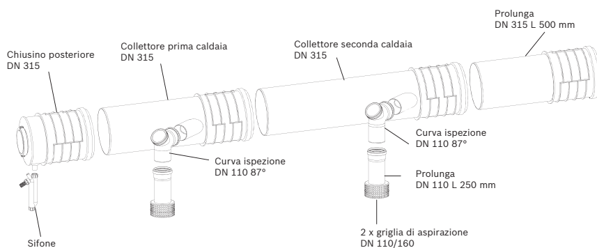
Estensione (ulteriore caldaia) per collettore combustivi Ø 315 mm
