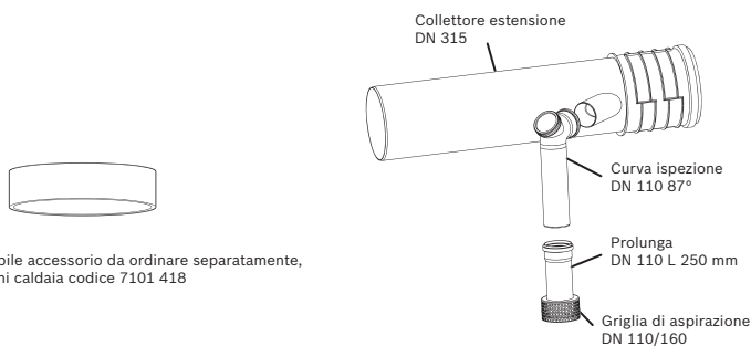
Estensione (ulteriore caldaia) per collettore combustivi Ø 315 mm
