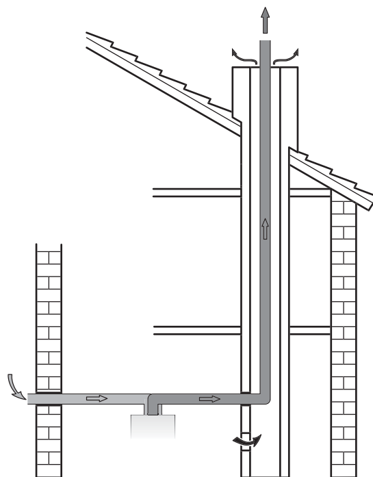
Tipologia di scarico "C53"
