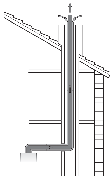
Tipologia di scarico "C33"
