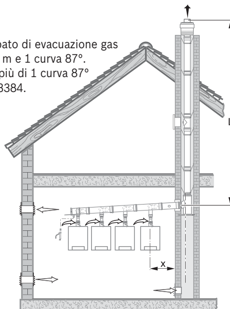
Lunghezze equivalenti indicative [m] di aspirazione ed evacuazione in depressione (es. verticale) per sistemi in cascata di CERAPURMAXX ZBR.-3 (1)
